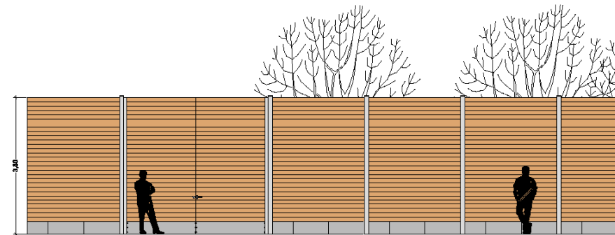
Lärmschutzwand Höhe 3,80m
