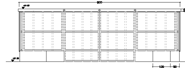
Schnitt A-A' 1:50
