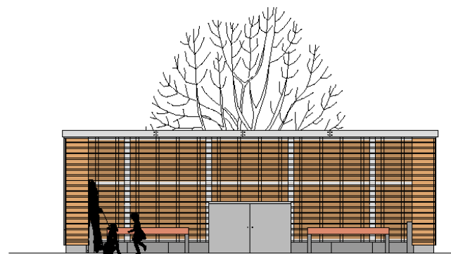
Unterstand Ansicht Süd-West M 1:50
