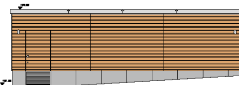
Geräteraum Ansicht Nord-West M 1:50
